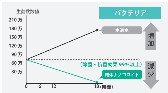
除菌・抗菌効果
